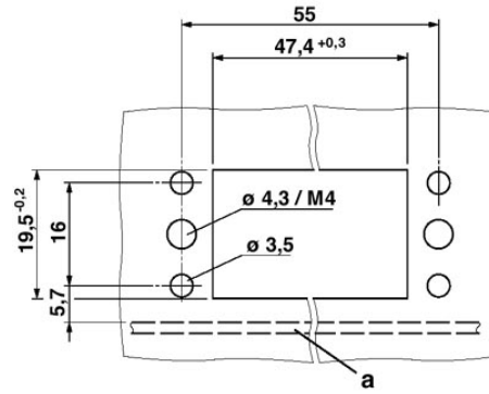
Szerelési kivágás
