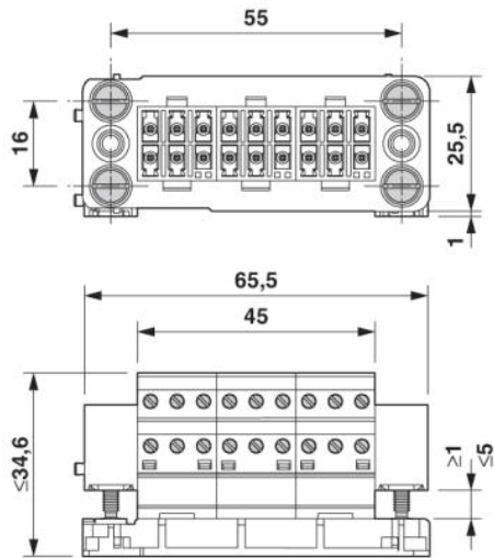
Érintkezőbetét
