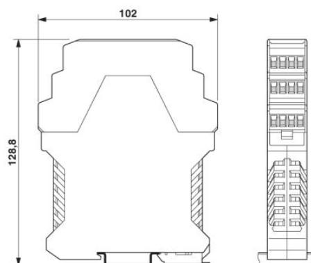
Disegno quotato del circuito stampato ME... utilizzando la parte superiore a tre piani
