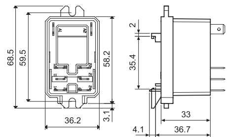
066.07 con relè
