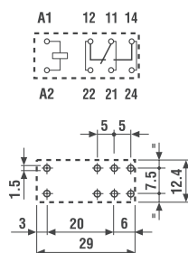
Vista lato rame
