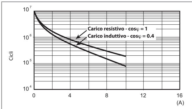
F 40 - Durata elettrica (AC) in funzione della corrente Tipi 40.11
