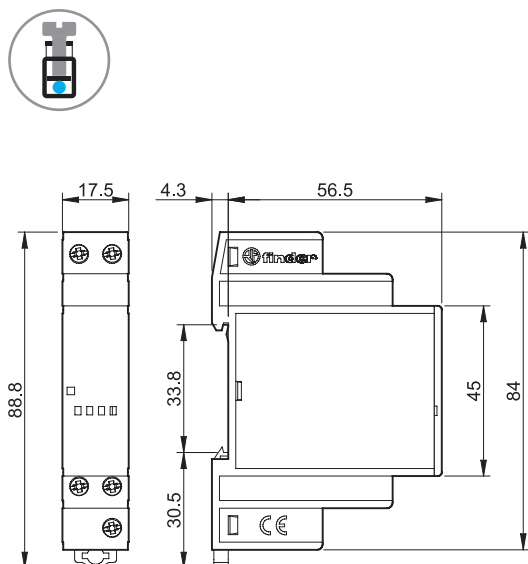
19.91 (modulo di potenza per 11.91) Morsetti a vite
