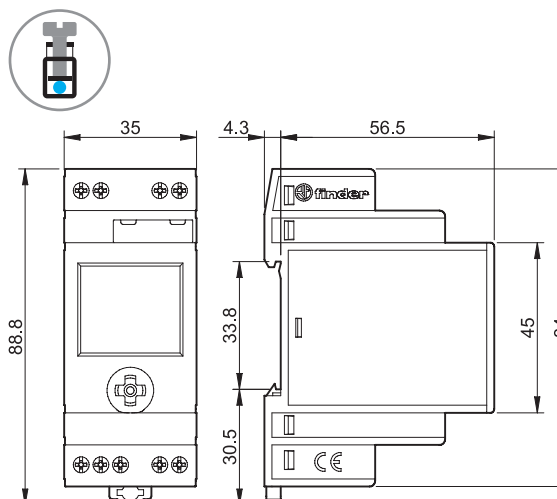
11.91 Morsetti a vite
