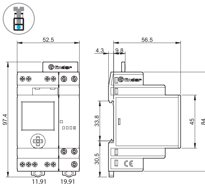
11.91 + Modulo di potenza 19.91 Morsetti a vite
