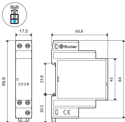
19.91 (modulo di potenza per 11.91) Morsetti a vite
