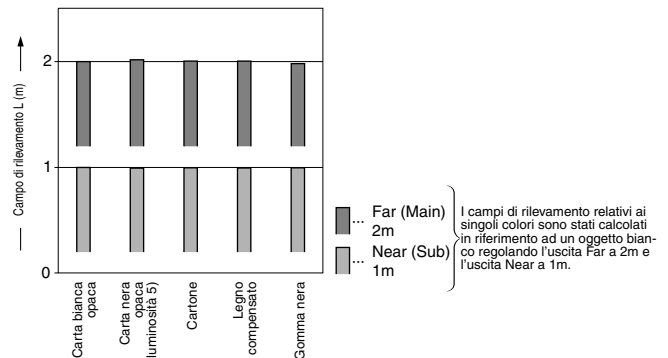
Correlazione colore dell'oggetto (200×200mm) - campo di rilevamento
