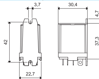
056.26 con relè
