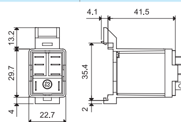
056.27 con relè
