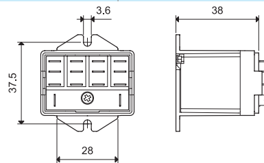
056.45 con relè
