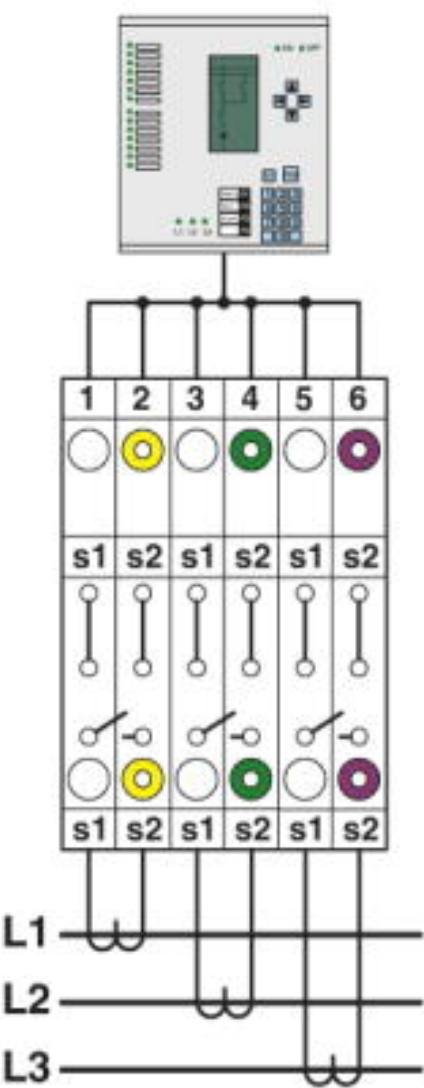
Convertitore trifase semplice
