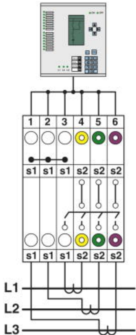
Convertitore trifase concatenato
