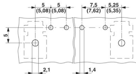
Preso base orizzontale
