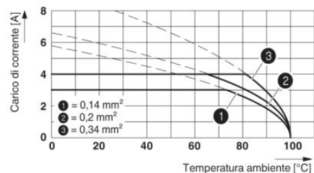
Tipo: FK-MC 0,5/...-ST-2,5 con MC 0,5/...-G-2,5
