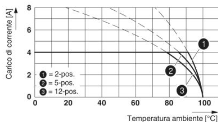
Tipo: FK-MC 0,5/...-ST-2,5 con MC 0,5/...-G-2,5
