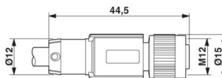
Connettore femmina M12 x 1, diritto
