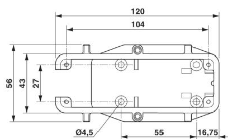
Disegno quotato vista dall'alto
