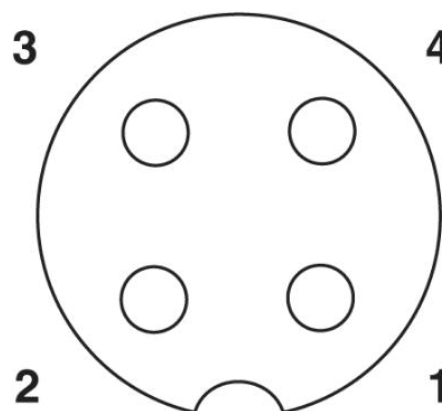
Pinning connettore femmina M12, 4 poli, codifica A, lato femmina
