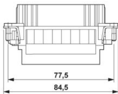
Disegno quotato
