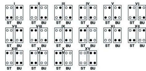
Codifica per alloggiamento con inserto portacontatti
