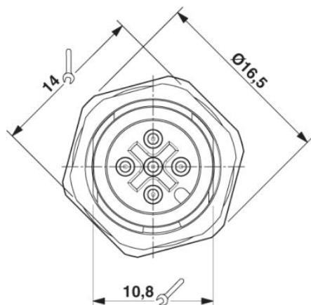
Disegno schema
