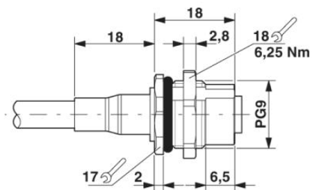
Passaparete M12
