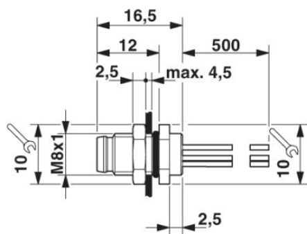
Connettore da incasso M8
