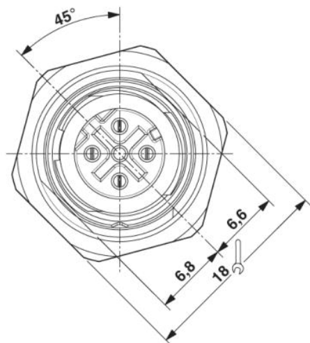
Disegno schema
