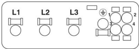
Pinning lato collegamenti
