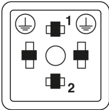
Pinning connettore per valvole, formato C
