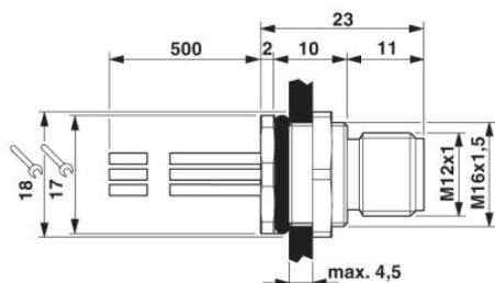
Conn. maschio da incasso M12
