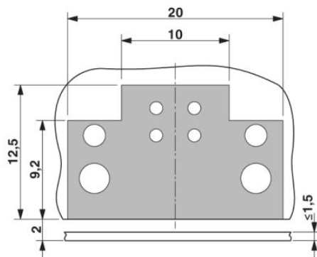
Superficie di bloccaggio sulla scheda c.s.
