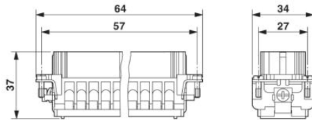
Inserto portacontatti femmina
