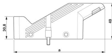
Disegno quotato, a=103,2
