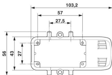
Disegno quotato vista dall'alto
