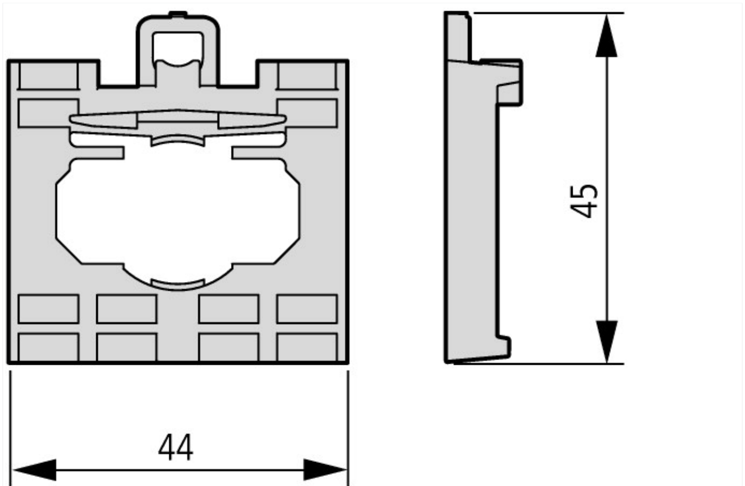
adattatore di fissaggio Adattatore di fissaggio (fissaggio frontale) per 4 elementi di contatto/LED
