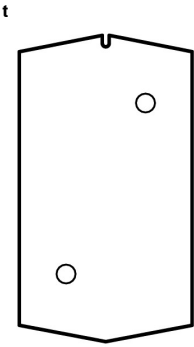
Parete retro: 2 X membrana passante fino a max. Ø 11 mm (non con CI-K2H)
