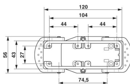
Disegno quotato, a=120
