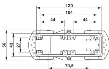
Disegno quotato vista dall'alto
