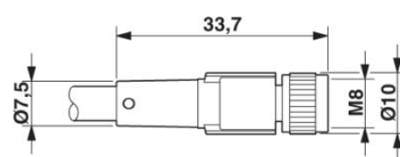
Connettore femmina M8 x 1, diritto
