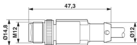
Connettore M12 x 1, diritto, schermato
