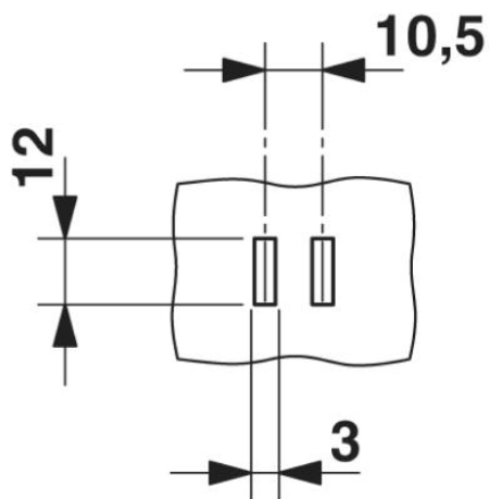
Dima di punzonatura
