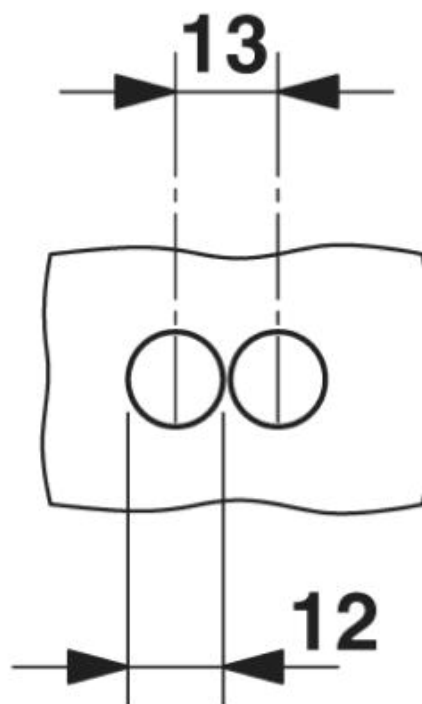
Dima di foratura
