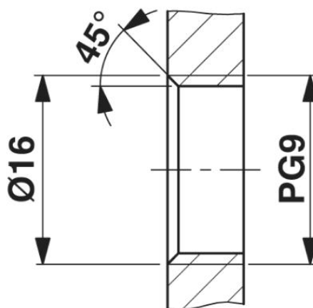
Sezione custodia per filettatura di fissaggio Pg9, montaggio a parete con filettatura
