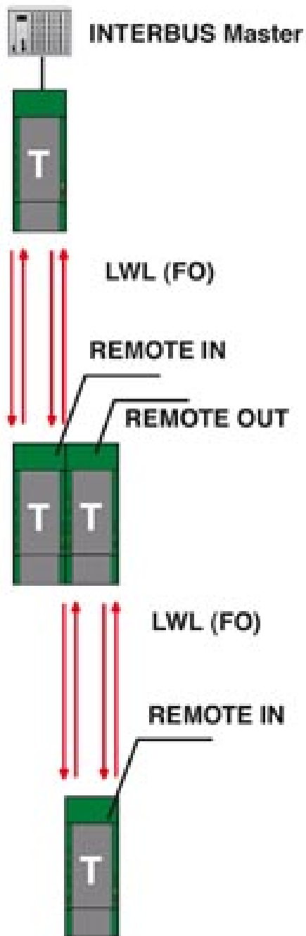
INTERBUS con collegamento ridondante PSI-MOS-RS-422
