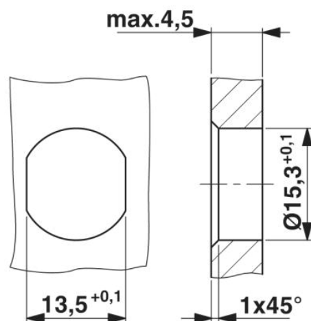
Sezione di montaggio con protezione antitorsione per filettatura Pg9
