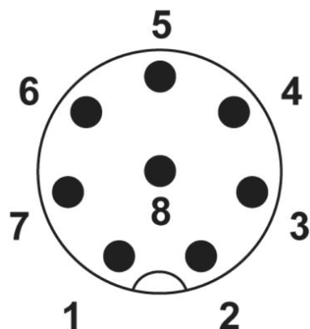
Pinning connettore M12, 8 poli, codifica A, lato maschio
