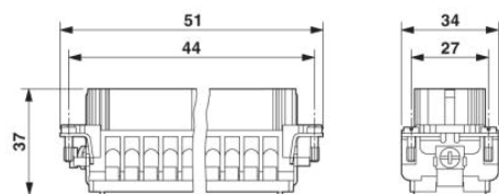
Inserto portacontatti femmina
