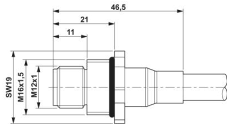
Conn. maschio da incasso M12
