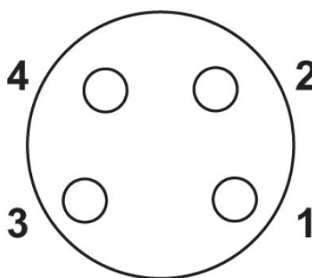
Pinning connettore femmina M8, 4 poli, vista lato femmina
