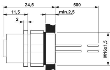
Connettore femmina da incasso M12, posizionabile
