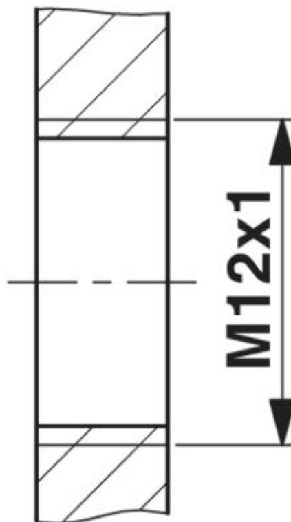
Sezione custodia per filettatura di fissaggio M12, montaggio a parete con filettatura
