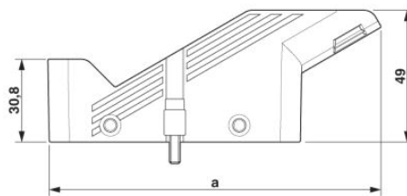
Disegno quotato, a=123,7
