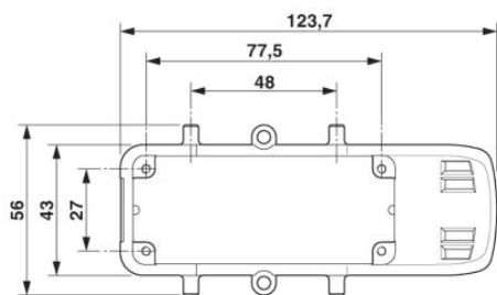
Disegno quotato vista dall'alto
