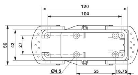
Disegno quotato vista dall'alto
