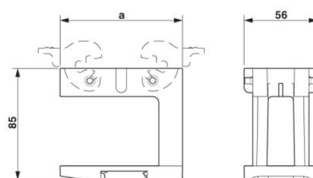
Disegno quotato, a=120
