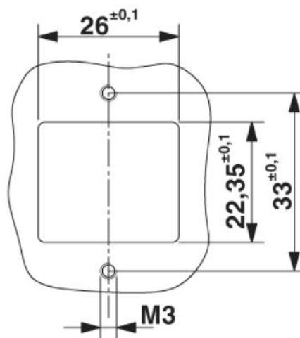
Dima di foratura:
