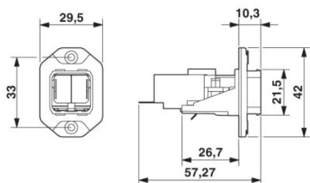
Telaio da incasso SCRJ Push-Pull
