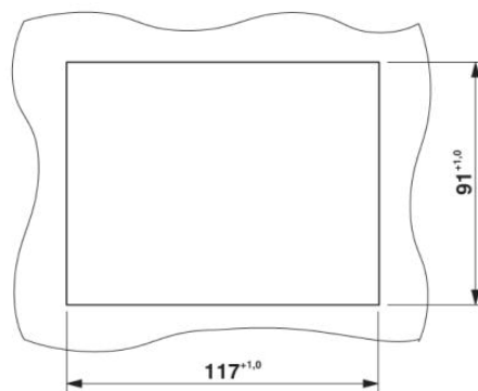
Dima di foratura:
