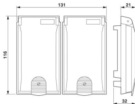
Telaio da incasso
