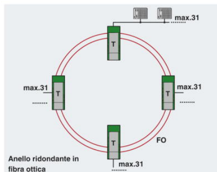
Anello ridondante in fibra ottica
