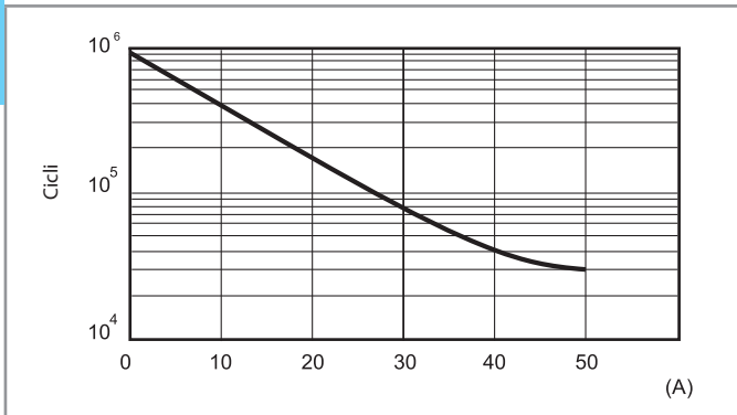
F 67 - Durata elettrica in funzione della corrente (carico AC1/AC7a)
