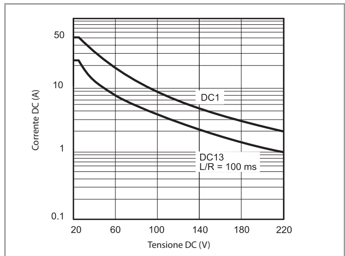
H 67 - Massimo potere di rottura su carichi in DC (67.xx-x500)
