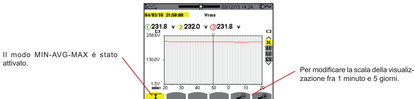
Figura 80: Vrms (3L) senza MIN-AVG-MAX
