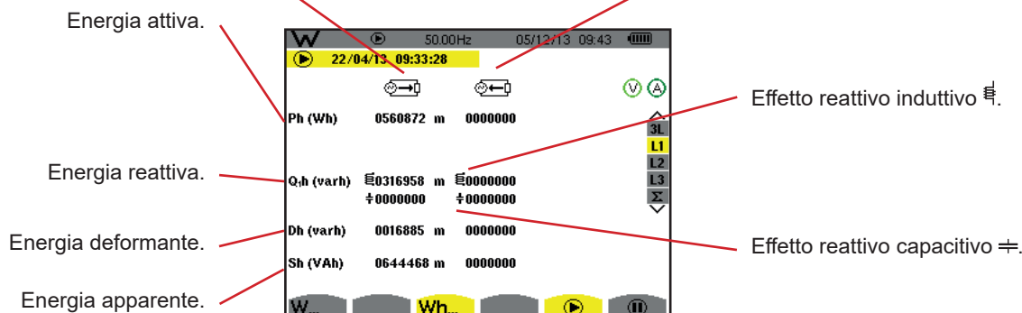
Figura 102: Lo schermo di visualizzazione delle energie consumate e generate in L1
