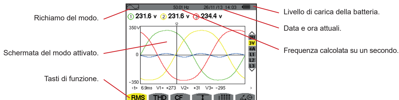
Figura 3: Esempio di schermo
