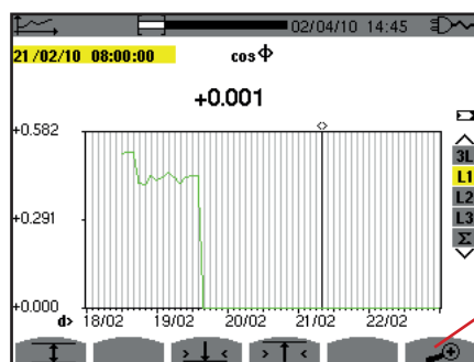
Figura 95: \cos \Phi (L1) caricamento / calcolo dei valori completo senza MIN-AVG-MAX per un collegamento trifase con neutro.
