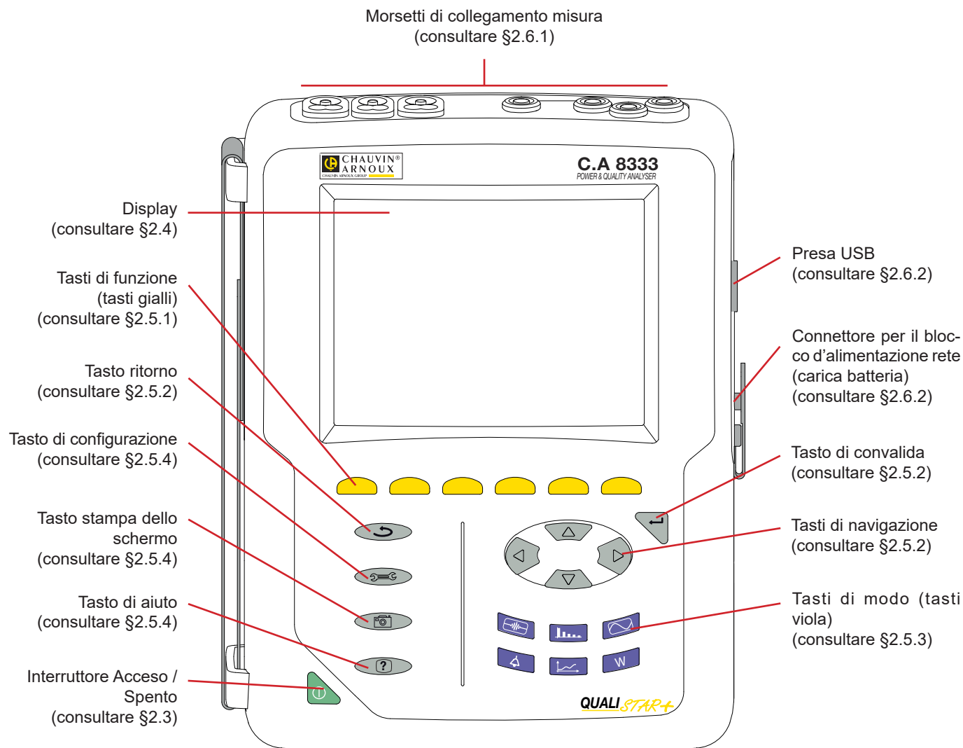
Figura 2: Vista generale del Qualistar+
