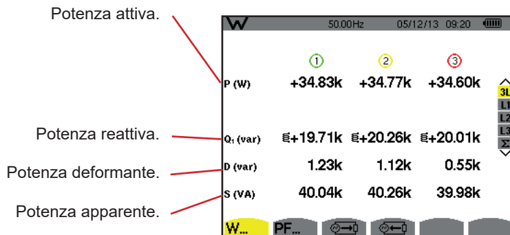
Figura 97: Lo schermo delle potenze in 3L.
