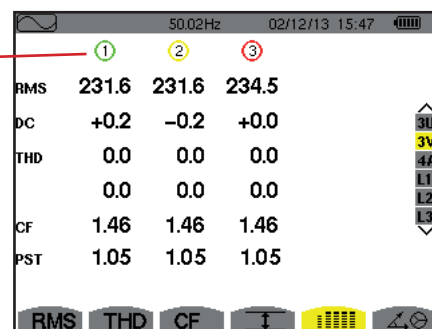
Figura 68: Lo schermo di visualizzazione simultanea in 3V
