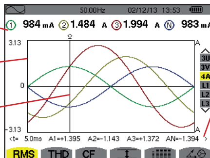
Figura 55: Lo schermo di visualizzazione RMS in 4A
