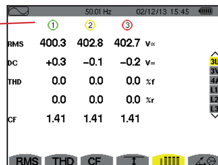
Figura 67: Lo schermo di visualizzazione simultanea in 3U
