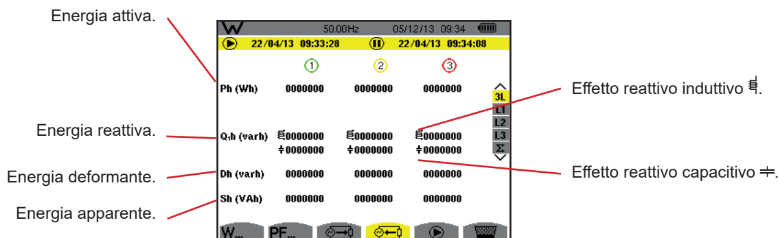
Figura 100: Lo schermo di visualizzazione delle energie generate in 3L
