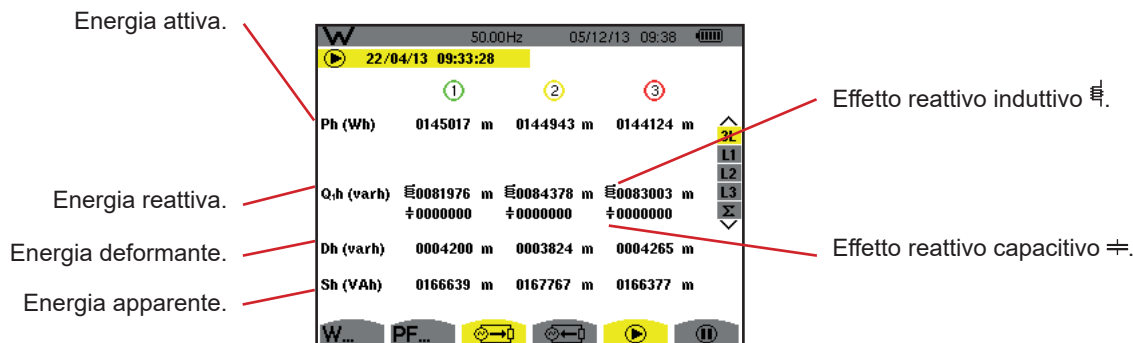
Figura 99: Lo schermo di visualizzazione delle energie consumate in 3L
