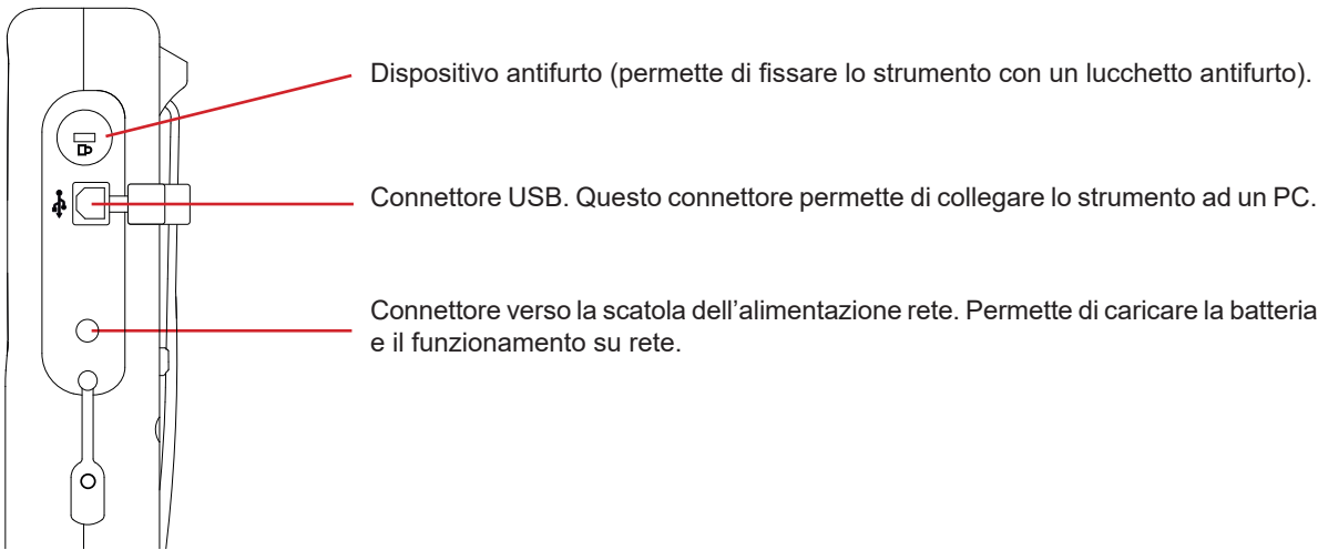
Figura 5: I connettori laterali
