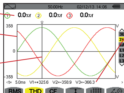
Figura 58: Lo schermo di visualizzazione THD in 3V
