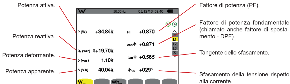
Figura 101: Lo schermo di visualizzazione delle potenze e delle grandezze associate in L1
