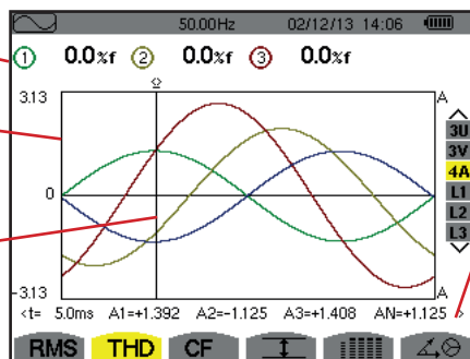
Figura 59: Lo schermo di visualizzazione THD in 4A
