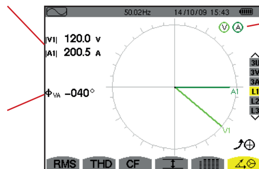
Figura 72: Lo schermo di visualizzazione del diagramma di Fresnel in L1
