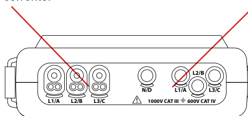
Figura 11: I morsetti di collegamento
