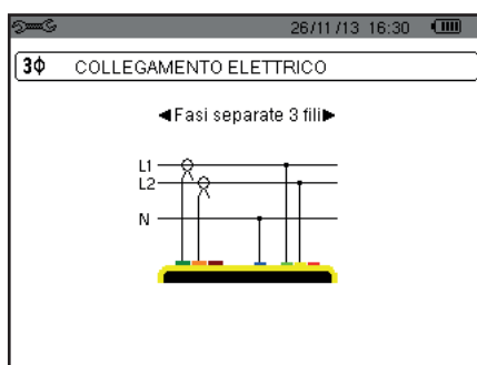
Figura 13: Collegamento in bifase a 3 fili
