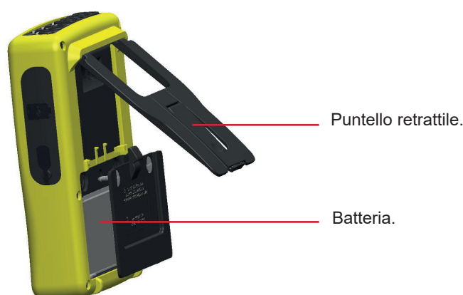
Figura 6: Puntello e sportello d'accesso alla batteria
