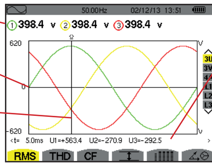
Figura 53: Lo schermo di visualizzazione RMS in 3U
