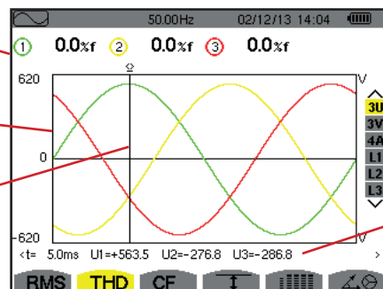
Figura 57: Lo schermo di visualizzazione THD in 3U
