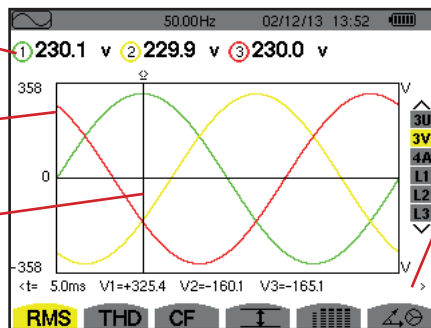
Figura 54: Lo schermo di visualizzazione RMS in 3V
