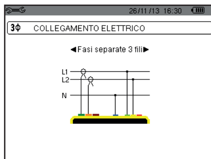
Figura 12: Collegamento in monofase a 2 fili
