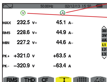
Figura 66: Lo schermo di visualizzazione Max-Min in L1
