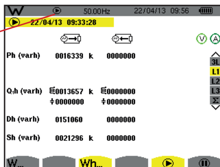
Figura 106: Lo schermo di conteggio d'energia in varh
