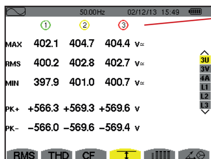
Figura 63: Lo schermo di visualizzazione Max-Min in 3U
