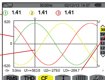
Figura 60: Lo schermo di visualizzazione CF in 3U
