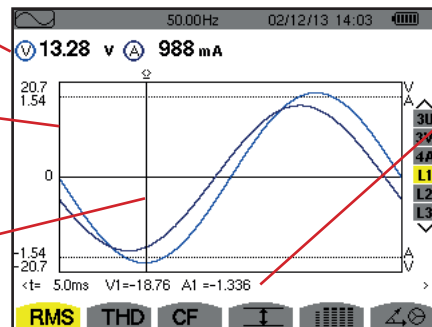
Figura 56: Lo schermo di visualizzazione RMS per L1
