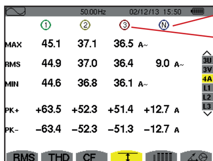
Figura 65: Lo schermo di visualizzazione Max-Min in 4A
