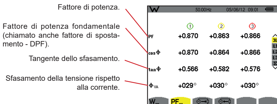
Figura 98: Lo schermo delle grandezze associate alle potenze in 3L.
