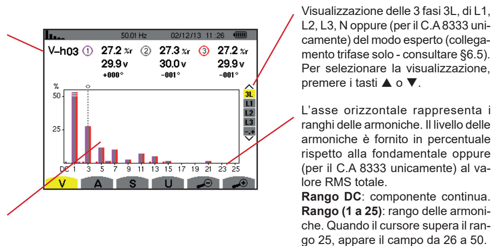
Figura 42: Esempio di visualizzazione delle armoniche della tensione semplice in 3L
