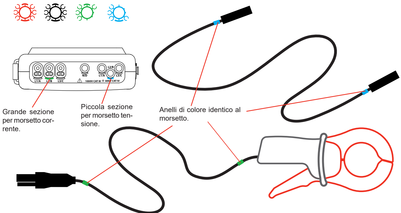
Figura 10: Identificazione dei cavi e dei morsetti
