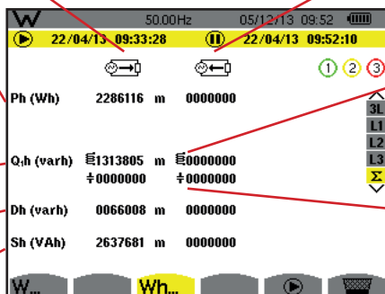
Figura 104: Lo schermo di visualizzazione delle energie consumate e generate totali in \Sigma
