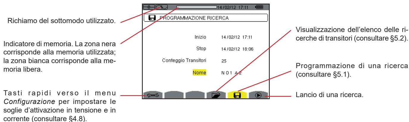
Figura 37: Lo schermo Programmazione di una ricerca in modo transitorio
