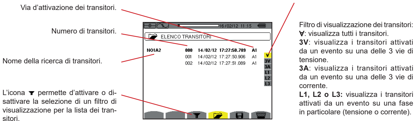
Figura 39: Lo schermo Elenco dei transitori in caso di un montaggio trifase a 4 fili
