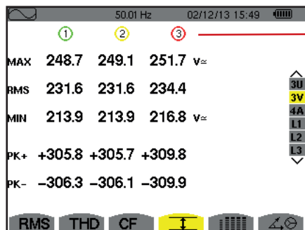
Figura 64: Lo schermo di visualizzazione Max-Min in 3V
