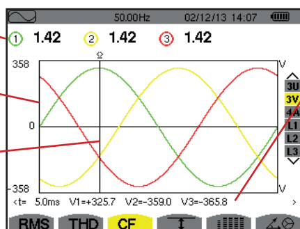
Figura 61: Lo schermo di visualizzazione CF in 3V
