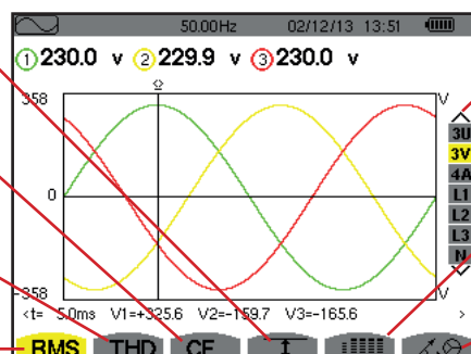
Figura 52: Lo schermo del modo Forme d'onda
