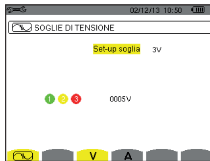
Figura 29: Lo schermo Soglie di tensione nel menu Modo transitorio
