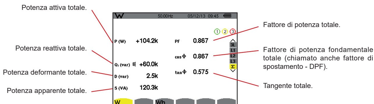
Figura 103: Lo schermo di visualizzazione delle potenze e delle grandezze totali associate in \Sigma
