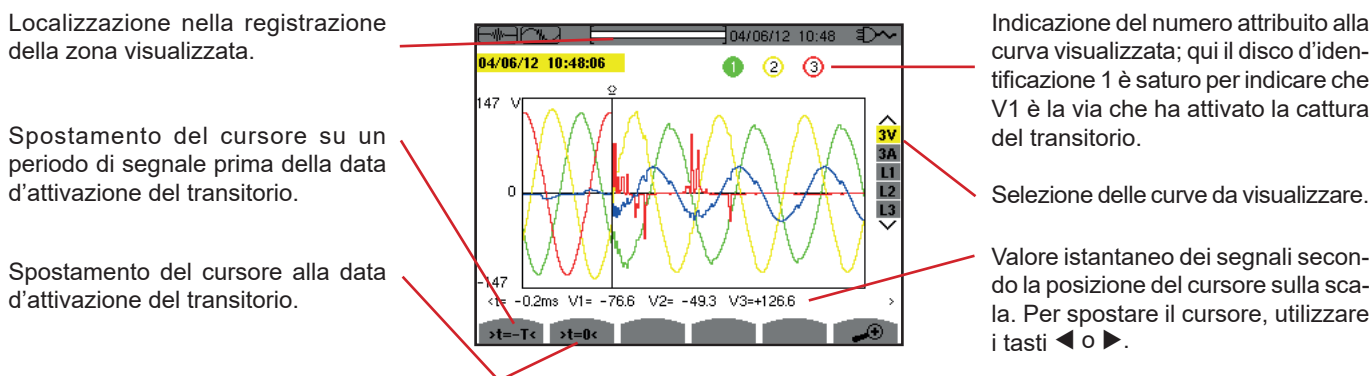
Figura 40: Esempio di visualizzazione dei transitori sotto forma di curve in collegamento trifase a 4 fili
