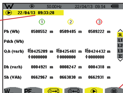
Figura 117: lo schermo d'avviamento del conteggio d'energia in Wh
