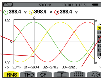
Figure 63: lo schermo di visualizzazione RMS in 3U
