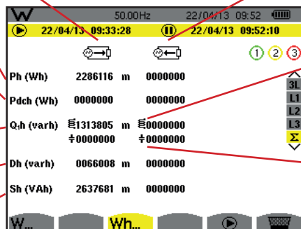
Figura 116: lo schermo di visualizzazione delle energie consumate e generate totali in \Sigma
